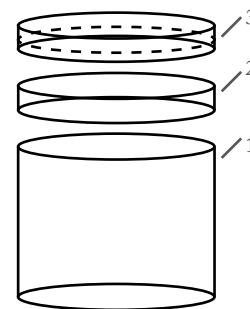
1 cilindro 20 L – 2 collare – 3 setaccio (griglia 20mm, 40mm, 60mm).
